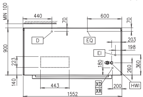
Felülnézet
